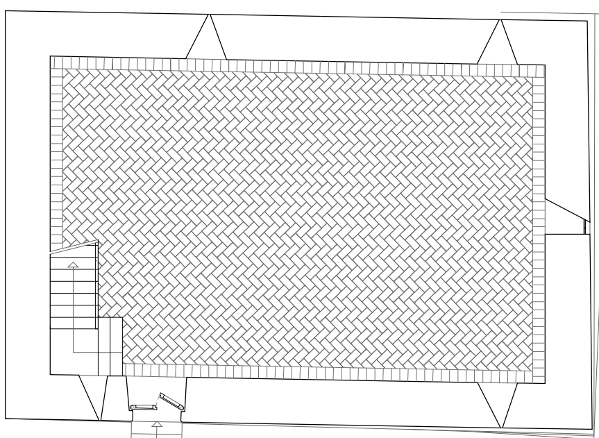
Planta de acceso (0.00 m)
