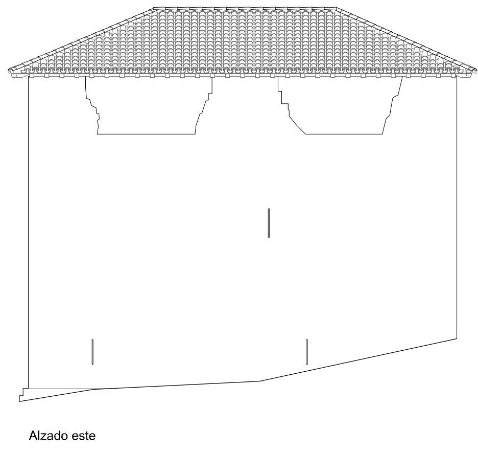
Alzado este
