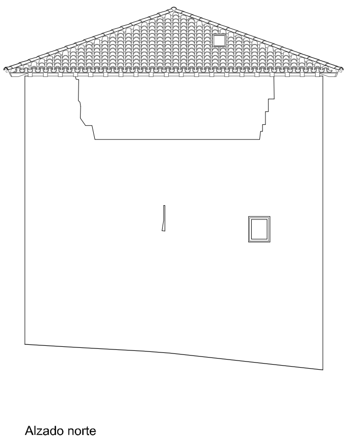
Alzado norte
