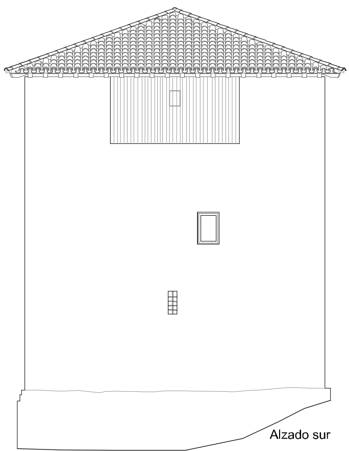
Alzado sur
