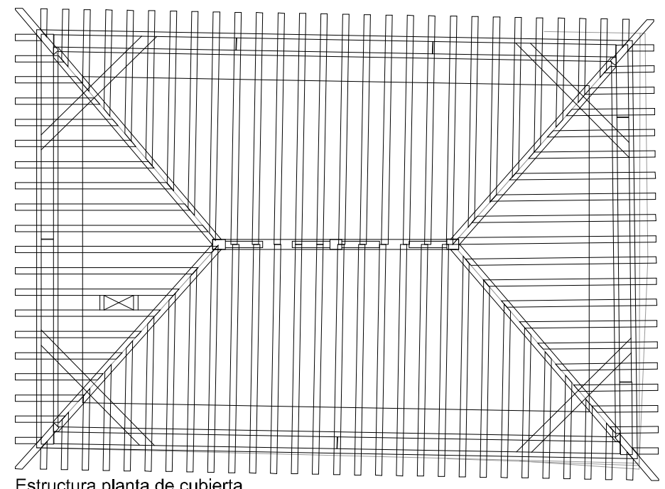
Estructura planta de cubierta
