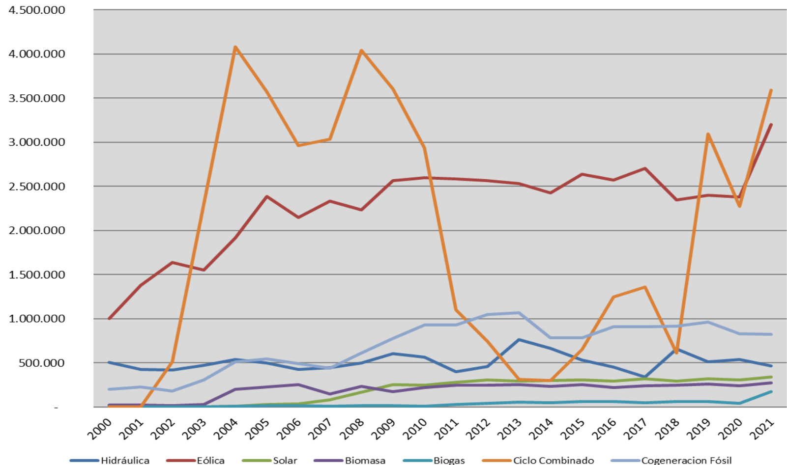
EVOLUCIÓN DE PRODUCCIÓN ELÉCTRICA POR TIPO DE GENERACIÓN DETALLADA
