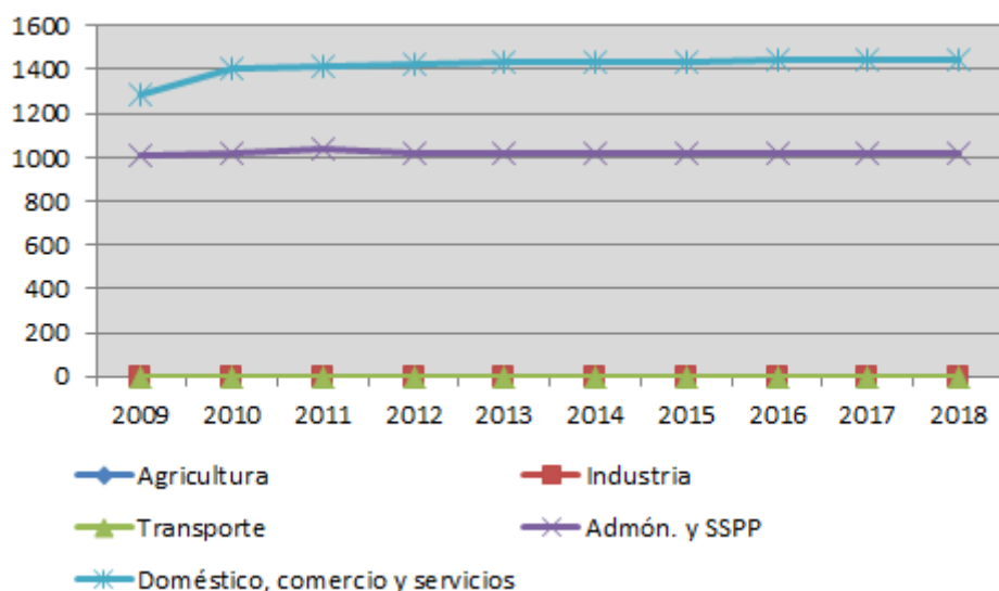
Gráfico 17. Consumo de solar térmica como energía final por sectores en Navarra 2009 a 2018 (TEP).
