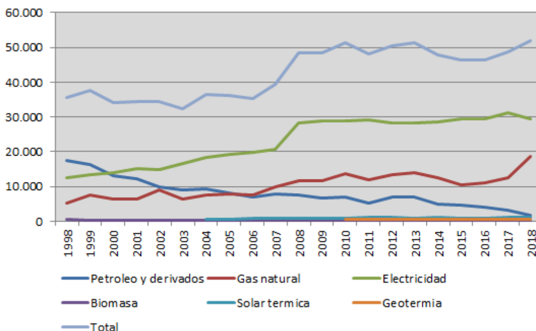
Gráfico 26. Evolución del consumo energía final de Administración y servicios públicos 1998-2018 (tep)
