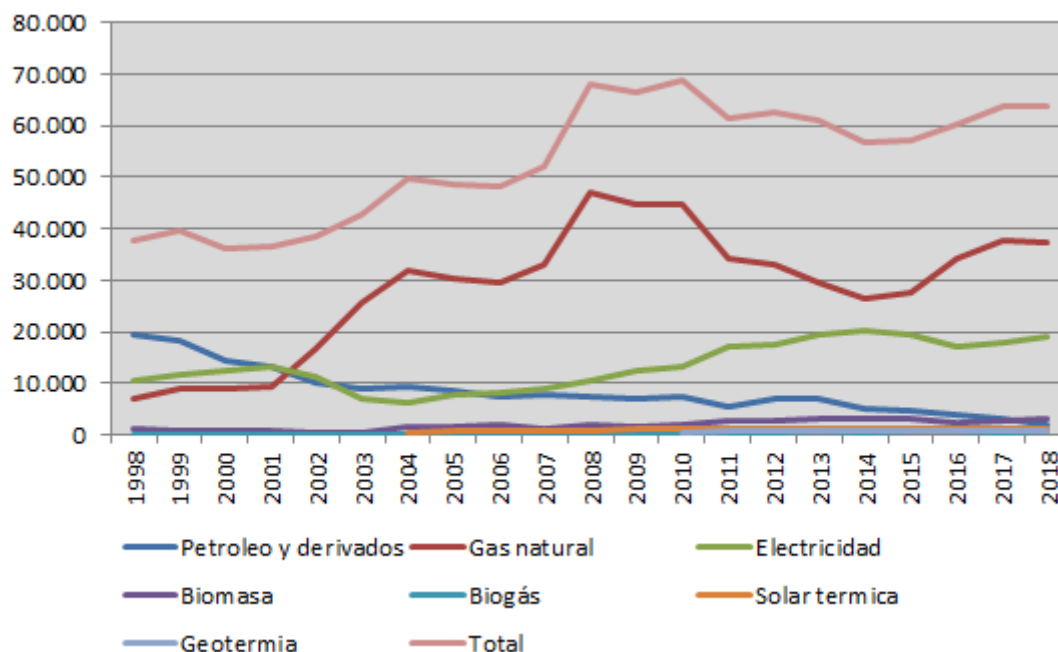
Gráfico 23. Variación de consumo energía primaria por tipo en Administración y servicios públicos en 1998-2018 (tep)
