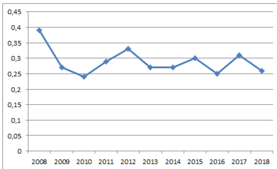
Gráfico 42. Evolución factor de emisión Mix nacional 2008 a 2018 (tm CO 2 /MWh)
