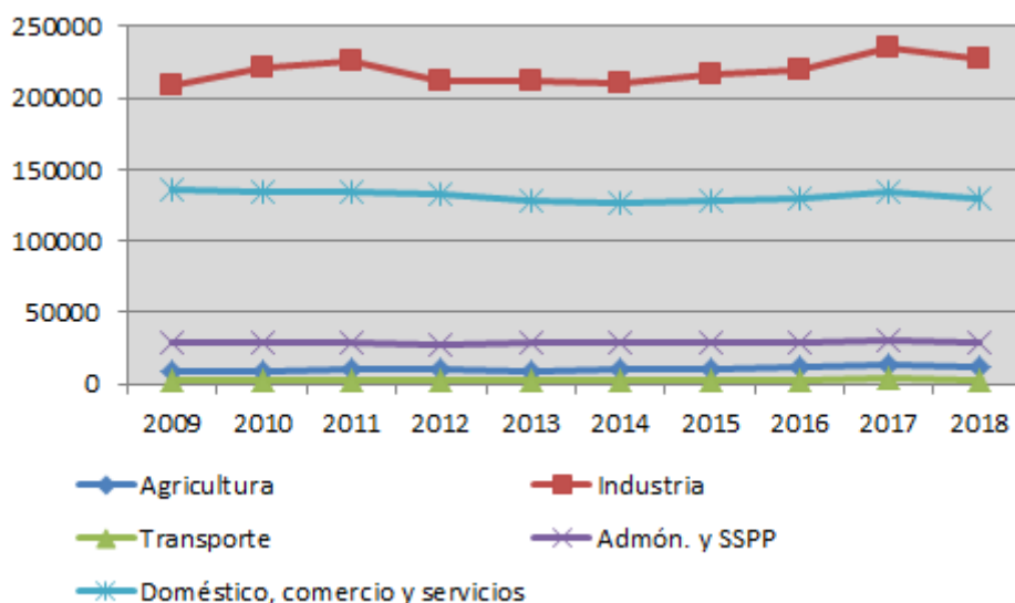
Gráfico 15. Consumo de electricidad como energía final por sectores en Navarra 2009 a 2018 (TEP).
