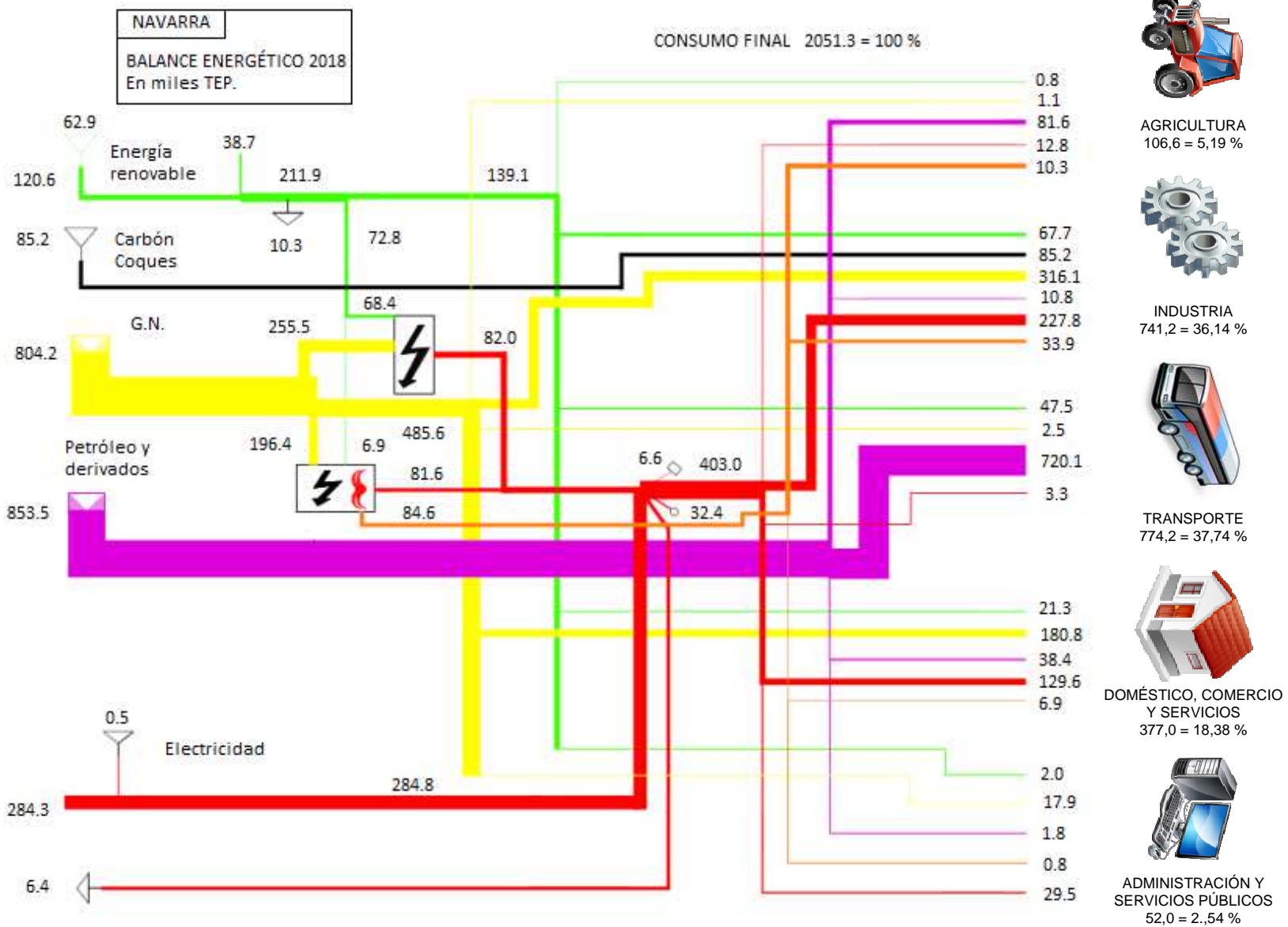
Figura 3. Representación gráfica del balance energético de Navarra 2018
