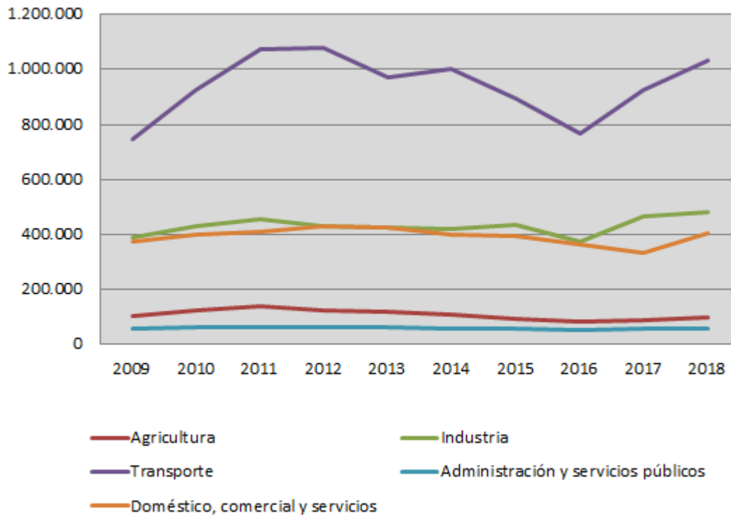
Gráfico 37. Evolución del coste de los combustibles empleados en el consumo de energía final en Navarra 2009-2018 por sectores (miles de euros corrientes).
