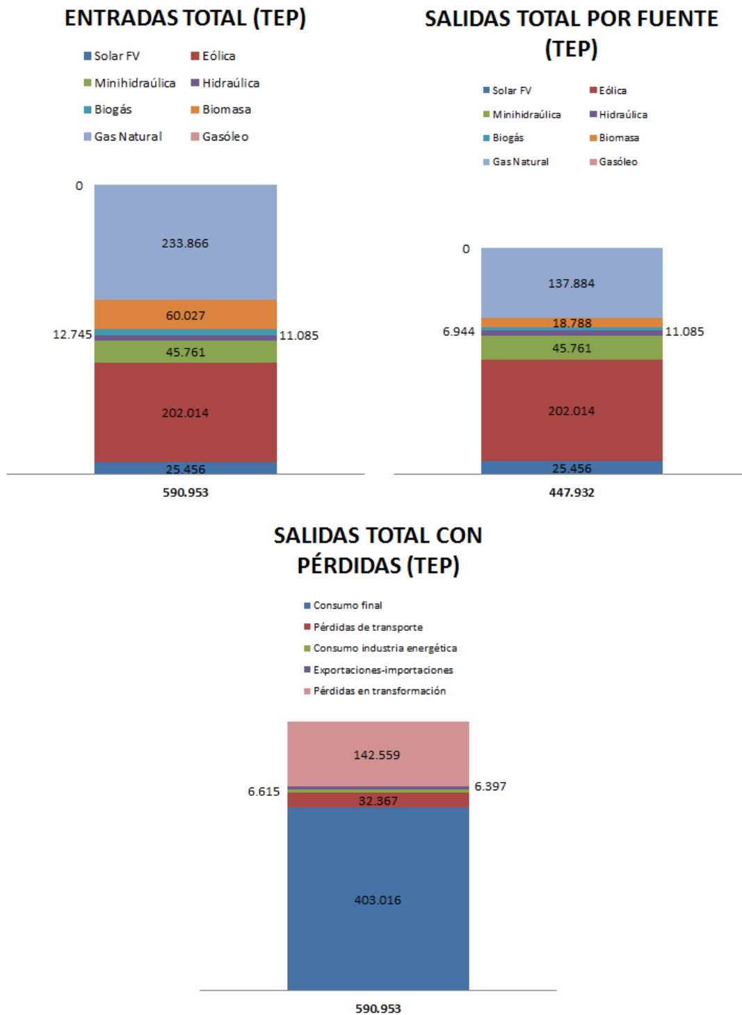
Gráfico 4. Generación eléctrica en Navarra en 2018 (TEP).
