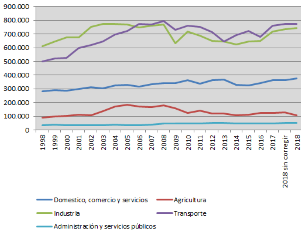
Gráfico 20. Consumo de energía final por sectores en Navarra 1998-2018 (TEP)
