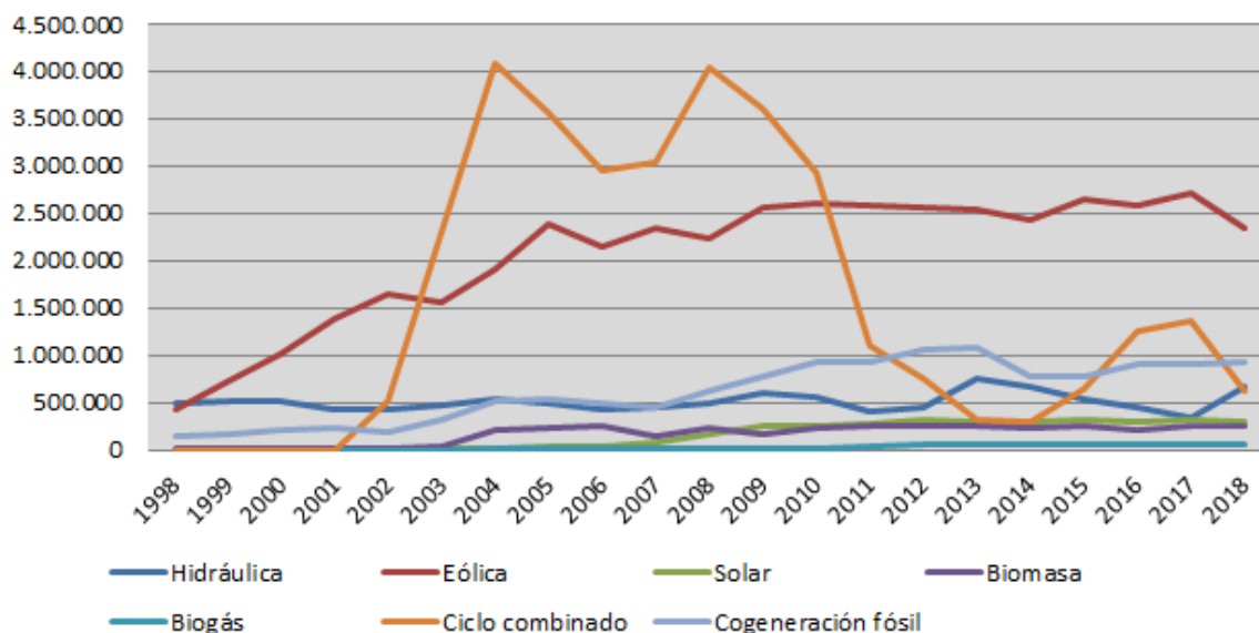
Gráfico 5. Producción eléctrica en Navarra 1998-2018 (MWh).
