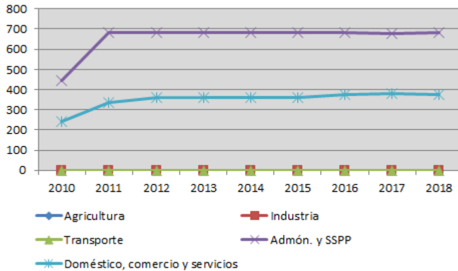
Gráfico 18. Consumo de geotermia como energía final por sectores en Navarra 2010 a 2018 (TEP).
