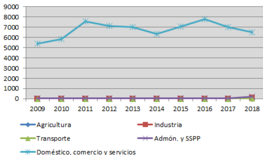
Gráfico 13. Consumo de GLP envasado como energía final por sectores en Navarra 2009 a 2018 (TEP).
