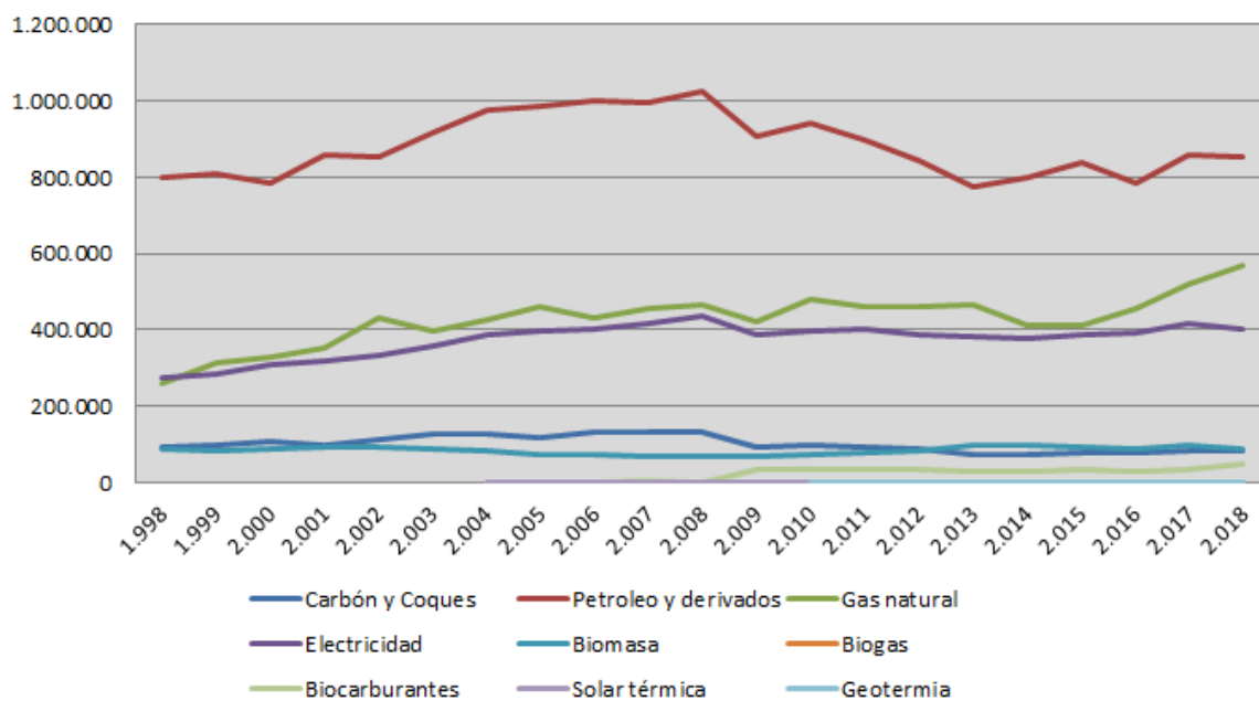
Gráfico 8. Consumo de energía final por tipo en Navarra 1998-2018 (TEP)
