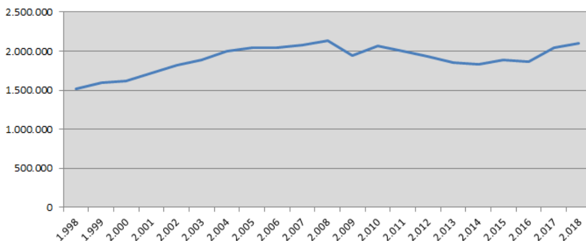
Gráfico 7. Consumo de energía final en Navarra 1998-2018 (TEP).
