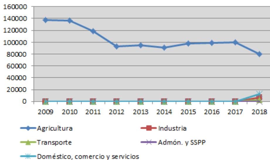
Gráfico 11. Consumo de gasóleo B como energía final por sectores en Navarra 2009 a 2018 (TEP).
