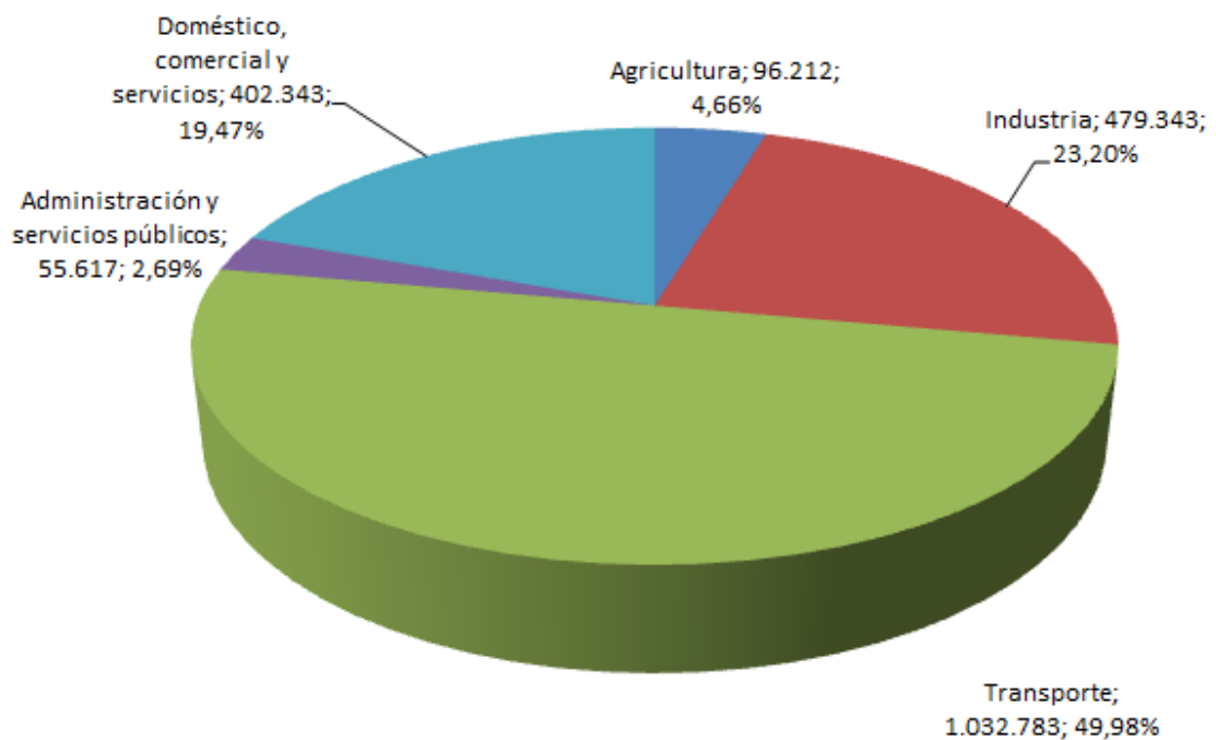
Gráfico 40. Coste de los combustibles empleados en el consumo de energía final en Navarra en 2018 por sectores (miles de euros y %)
