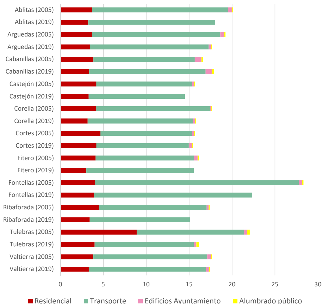
Figura 6 Evolución de los consumos por habitante (MWh/hab)
