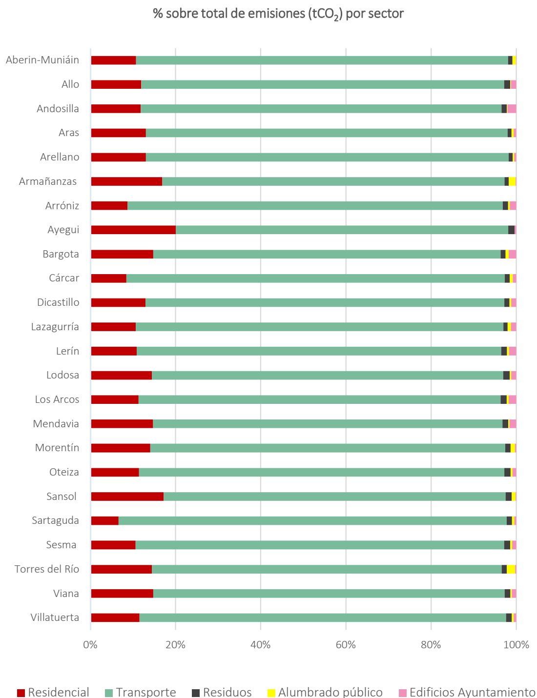
Figura 16 Distribución de emisiones (tCO 2 ) por sector sobre total del municipio, 2019
