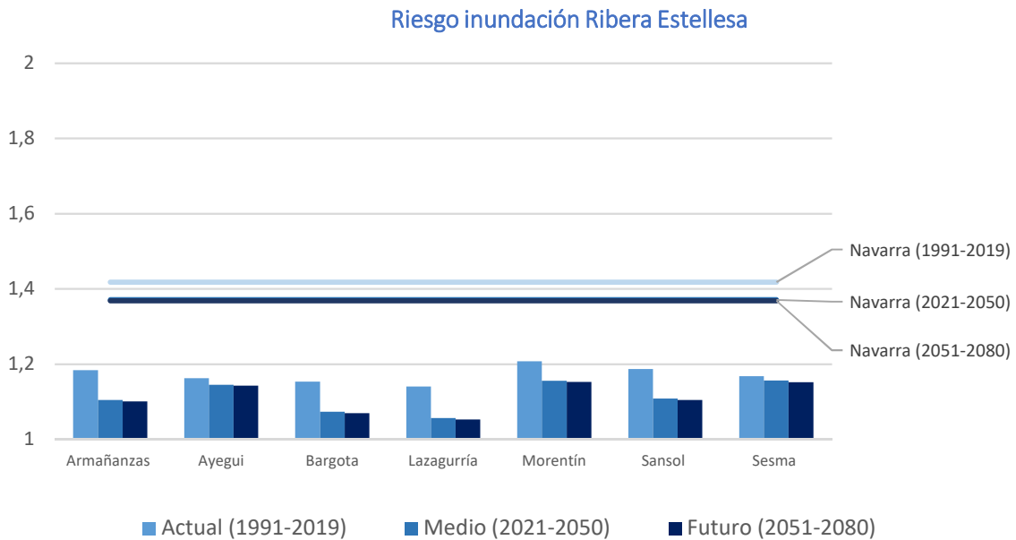
Figura 22 Evolución del riesgo frente a inundaciones
