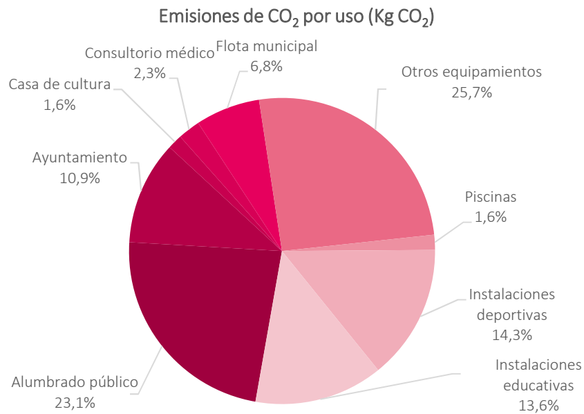
Figura 18 Emisiones municipales (kgCO 2 ) de la agrupación, % por uso
