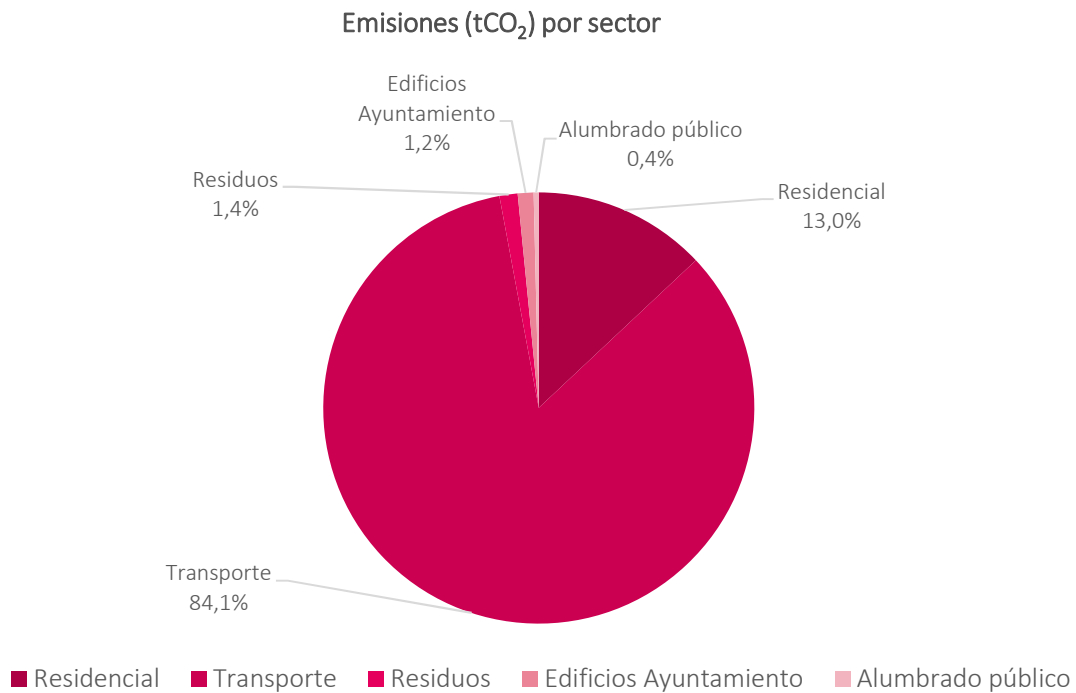
Figura 17 Emisiones (tCO 2 ) de la agrupación, por sector
