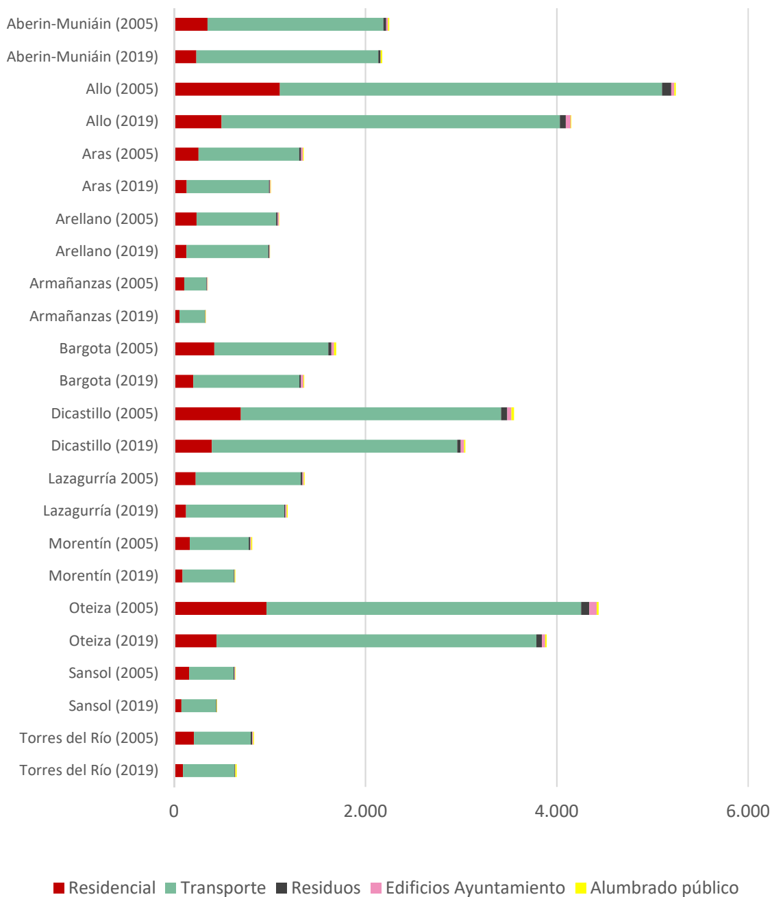
Figura 12 Evolución de las emisiones (tCO 2 ) por municipio y sector, para municipios <1.000 habitantes
