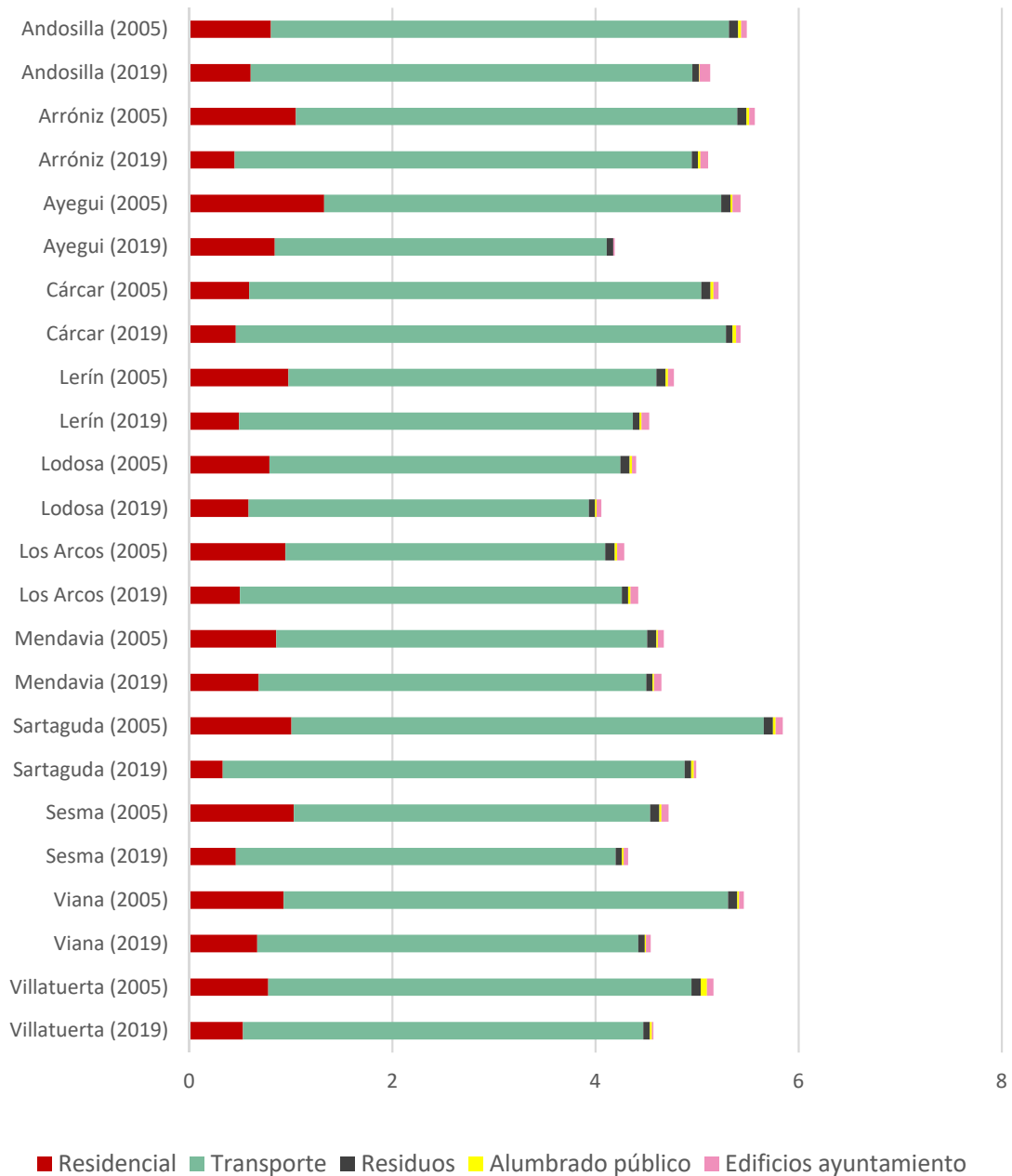
Figura 15 Evolución de las emisiones por habitante (tCO 2 /hab.), por municipio de >1.000 habitantes
