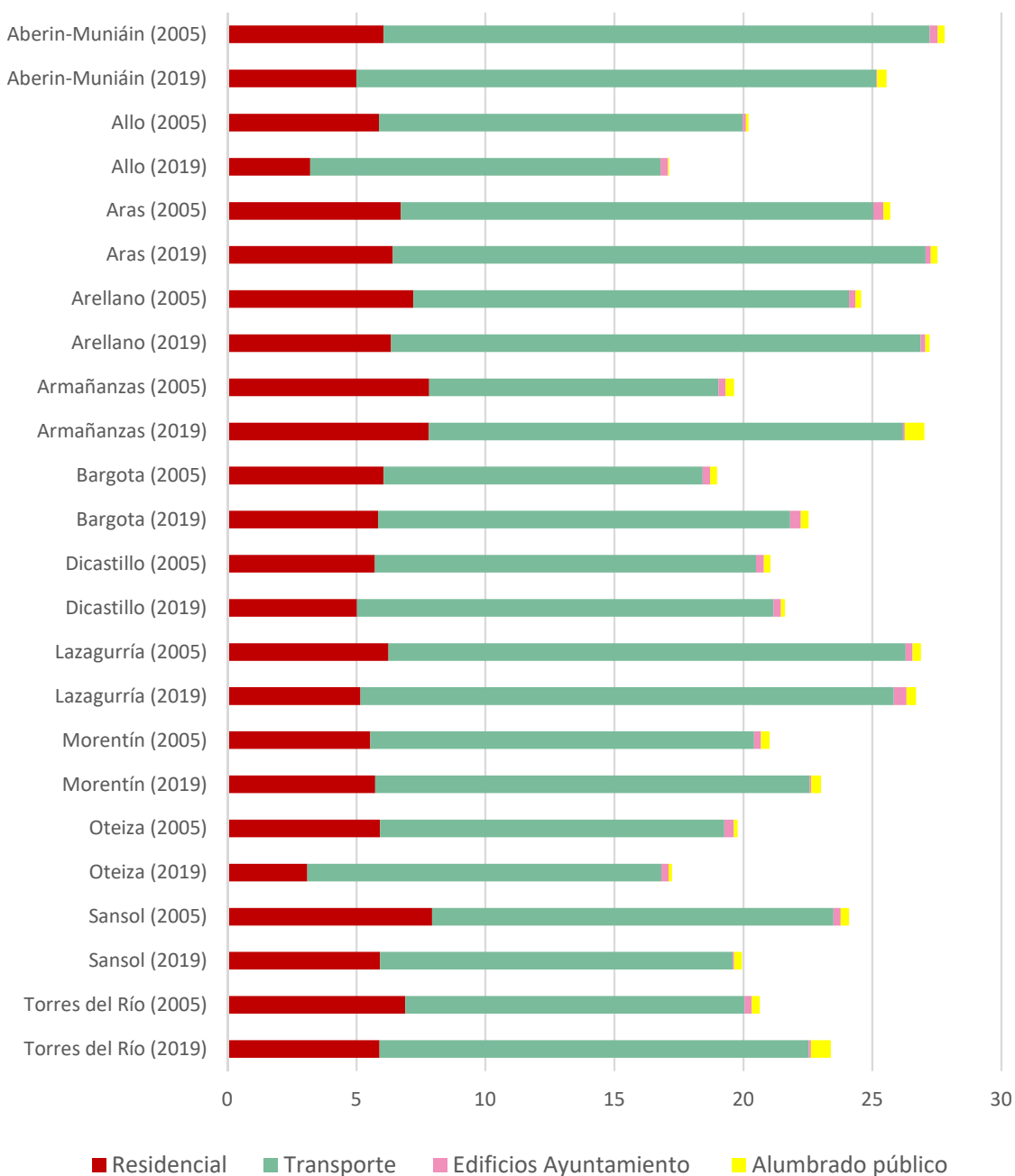
Figura 7 Evolución de los consumos por habitante (MWh/hab) para municipios <1.000 habitantes.
