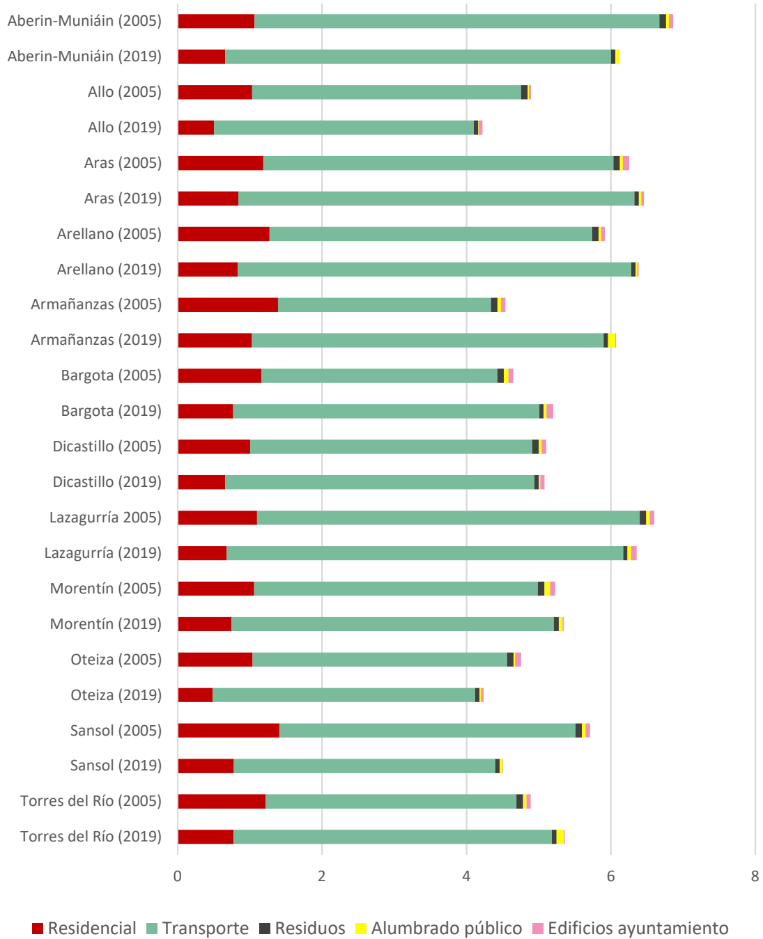
Figura 14 Evolución de las emisiones por habitante (tCO 2 /hab.), por municipio de <1.000 habitantes
