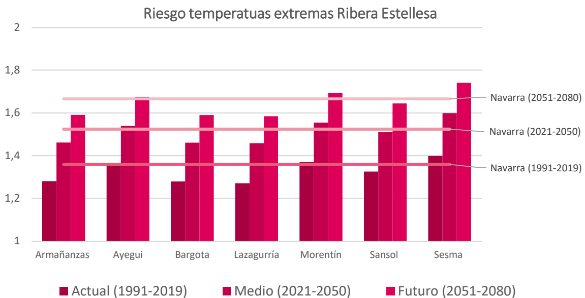
Figura 24 Evolución del riesgo frente a temperaturas extremas
