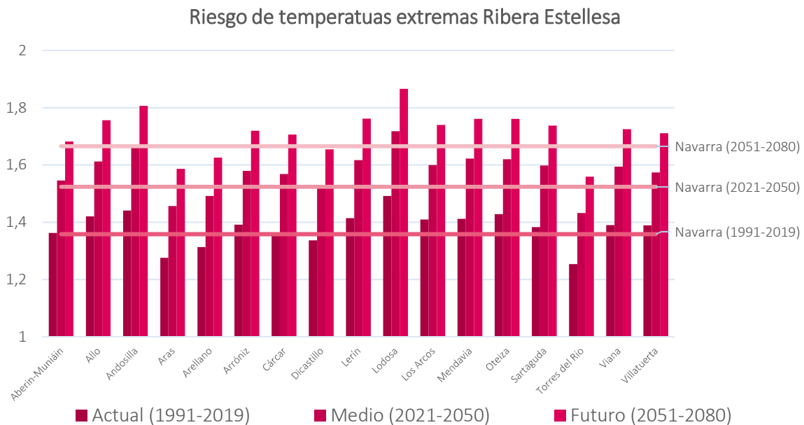
Figura 23 Evolución del riesgo frente a temperaturas extremas
