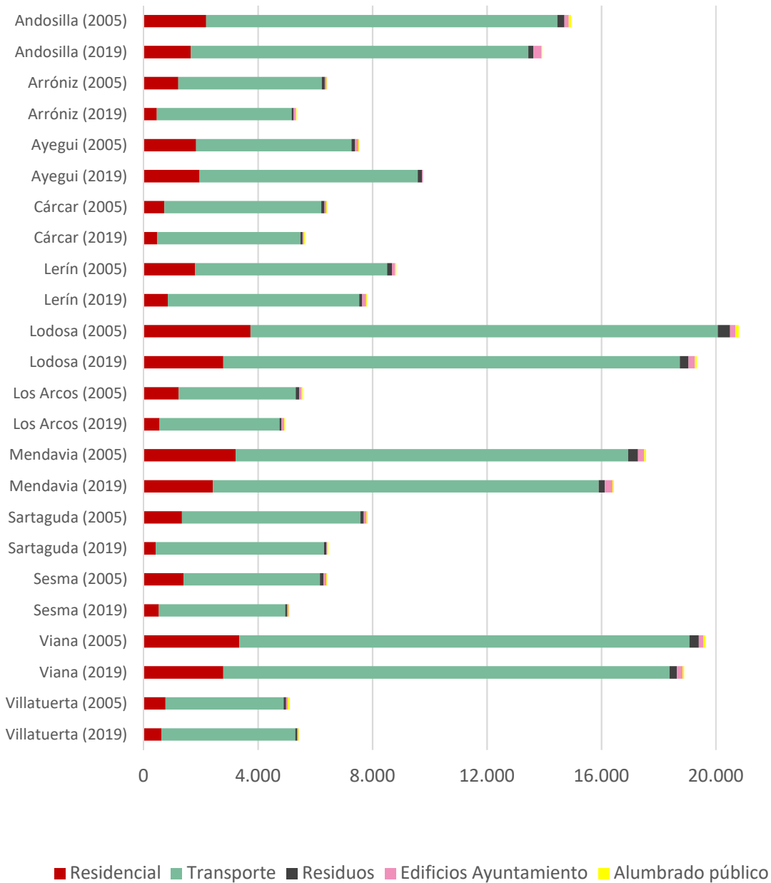
Figura 13 Evolución de las emisiones (tCO 2 ) por municipio y sector, para municipios >1.000 habitantes
