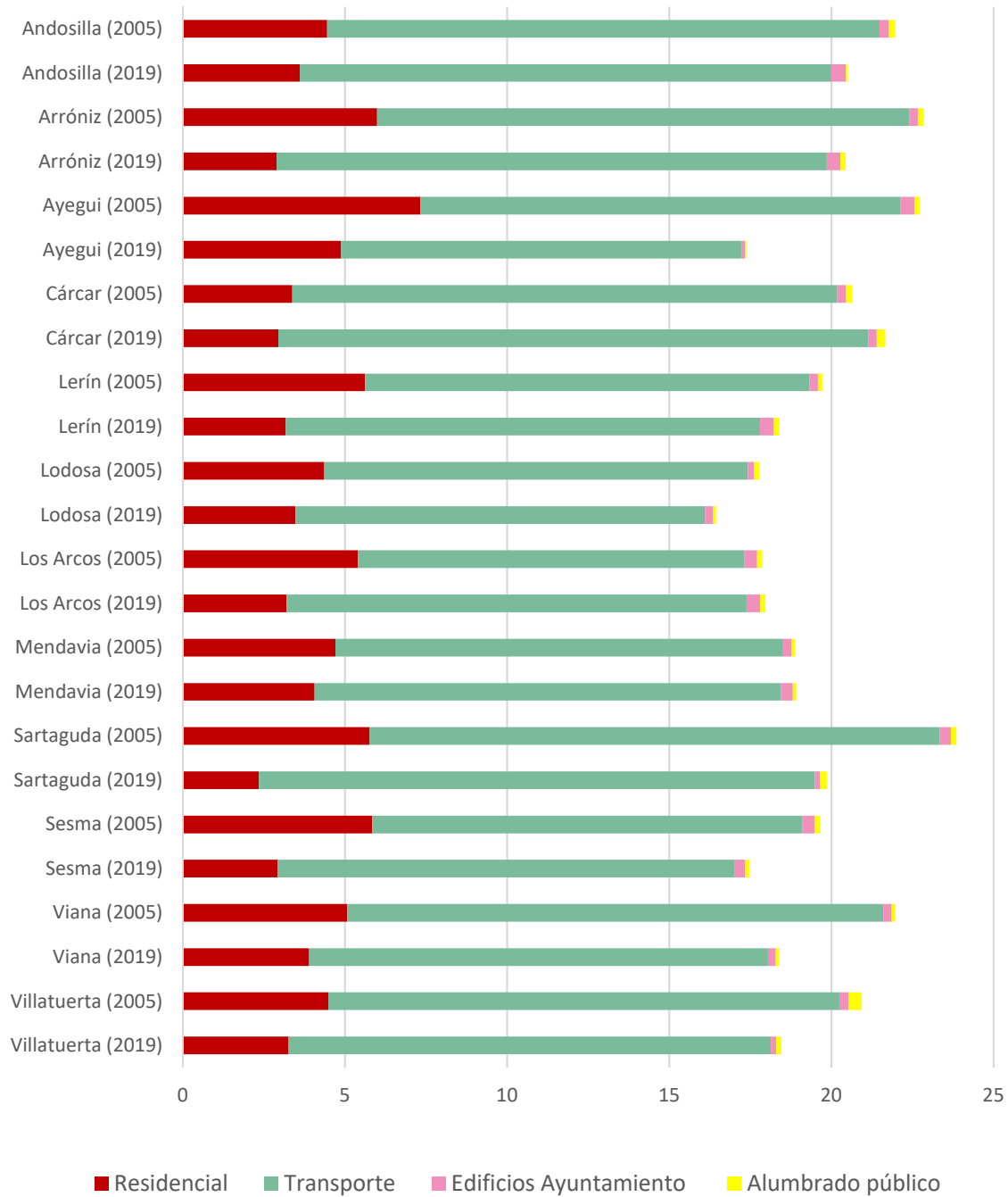
Figura 6 Evolución de los consumos por habitante (MWh/hab) para municipios >1.000 habitantes
