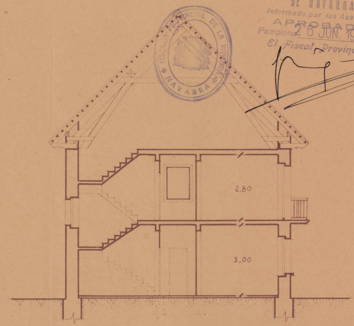
Sección A-B.
