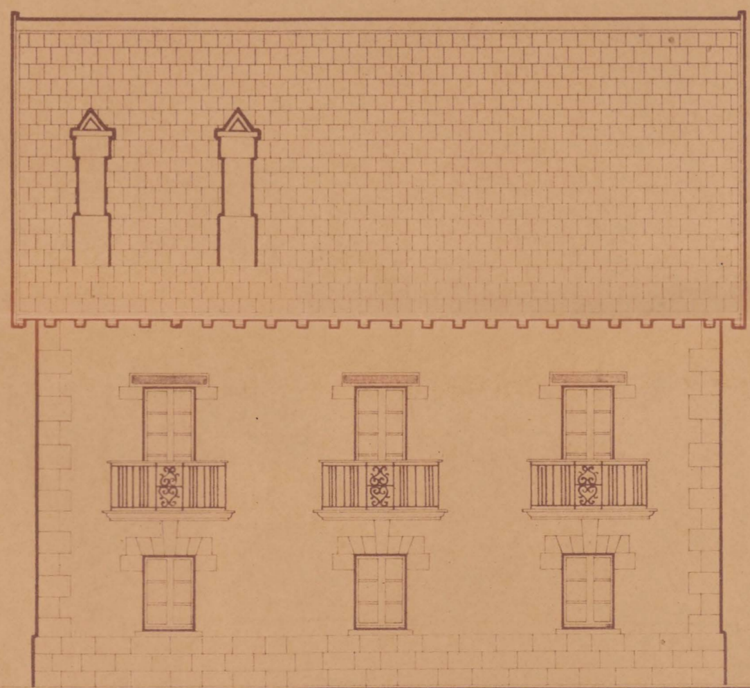
Fachada ltral.
