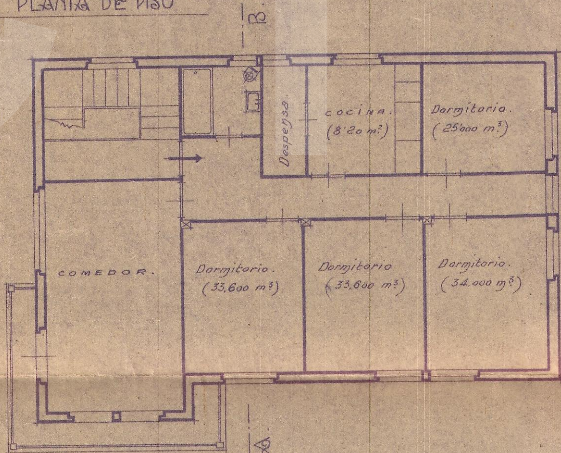
PLANTA DE PISO
