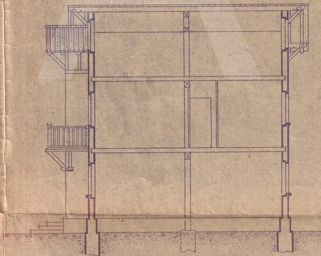
SECCION A.B.
