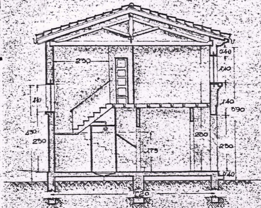
Sección a-b.
