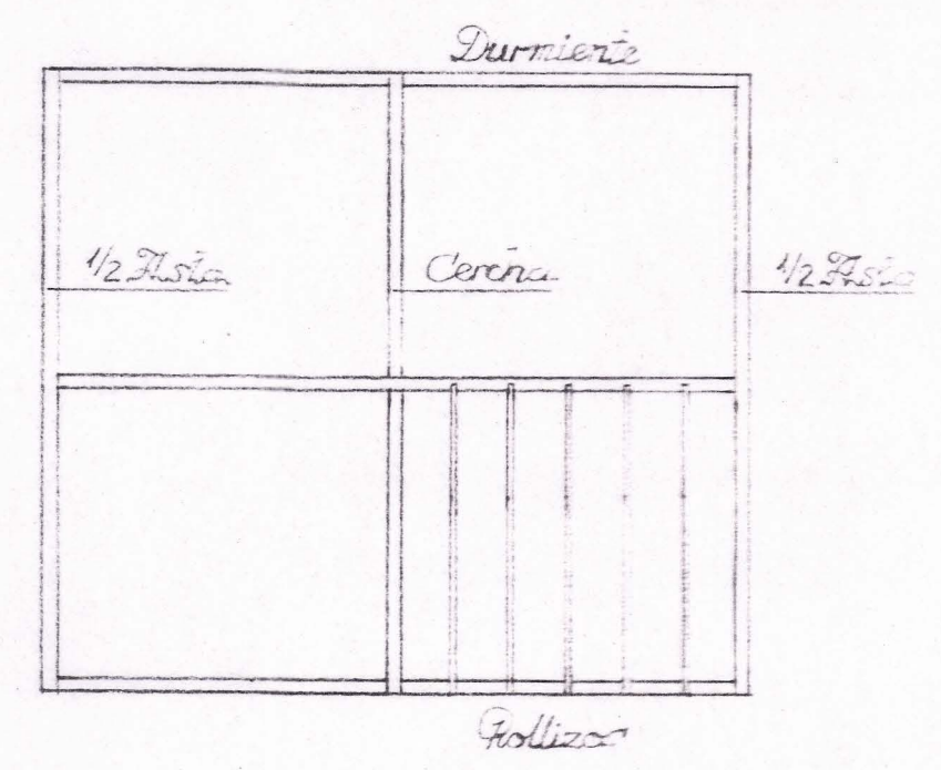
Estructura cubierta
