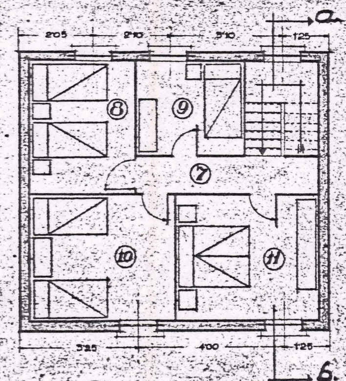
Planta primera.
