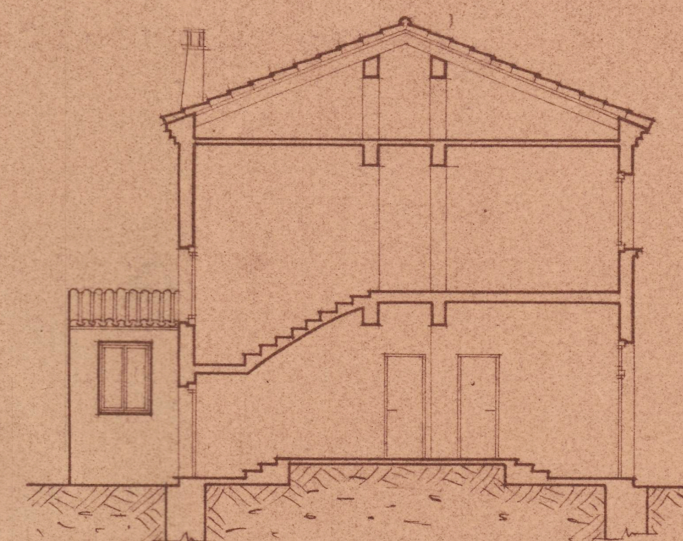
SECCION
