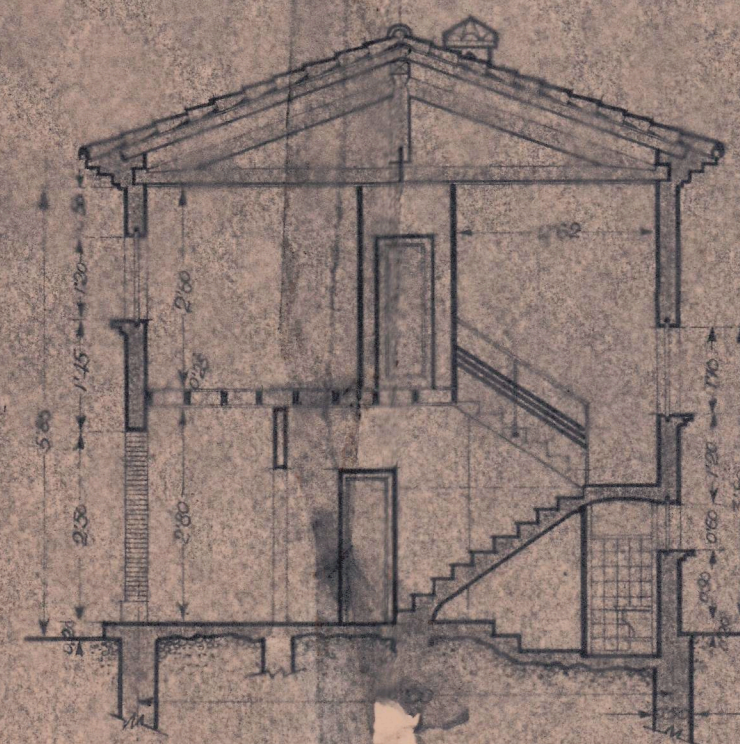
Sección a-b
