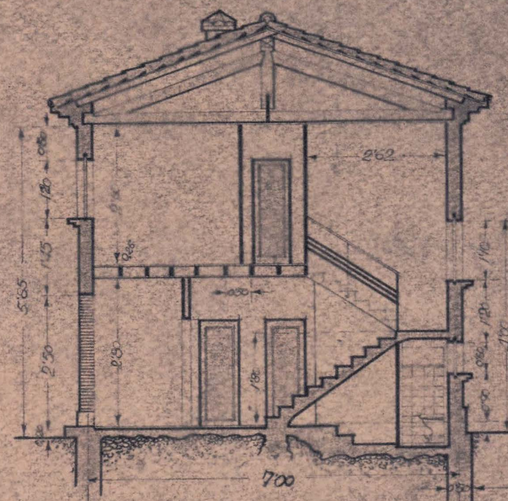
Seccion a - b
