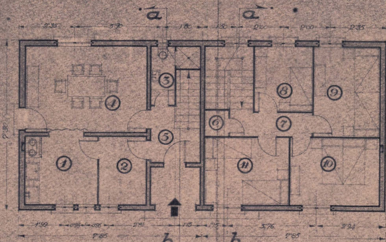
Plantas baja y primera
