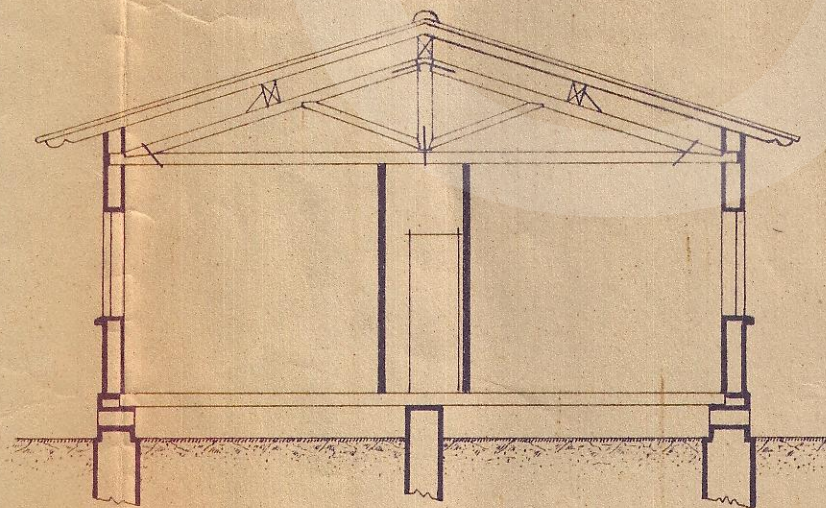
SECCION
