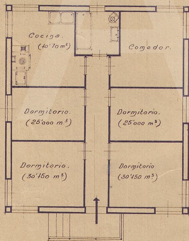
PLANTA
