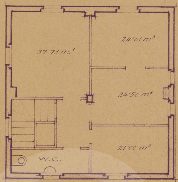
Planta principal
