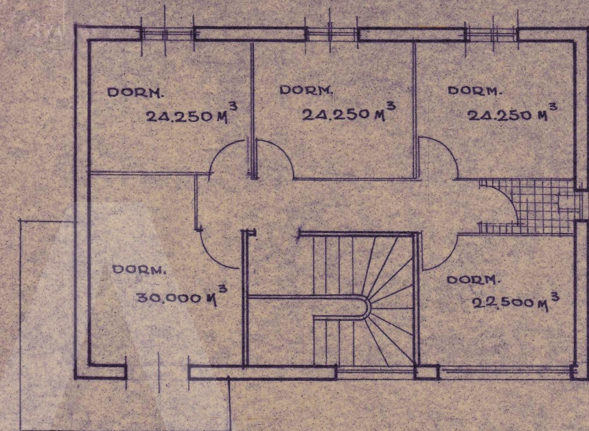
PLANTA PRAL.
