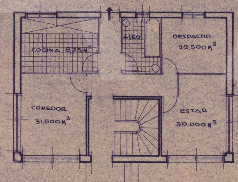
PLANTA BAJA
