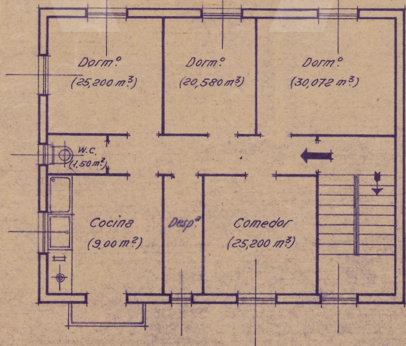
- PLANTA DEL PISO -
