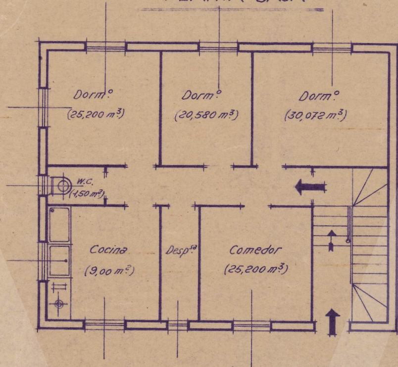
- PLANTA BAJA -
