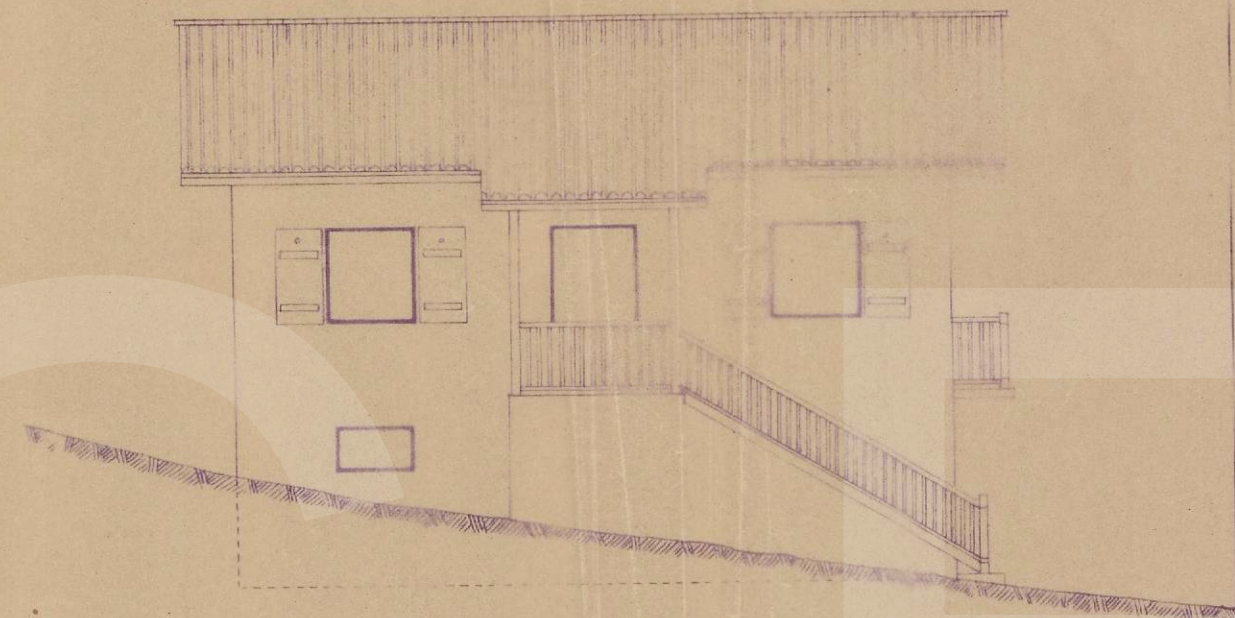
FACHADA LATERAL IZD.
