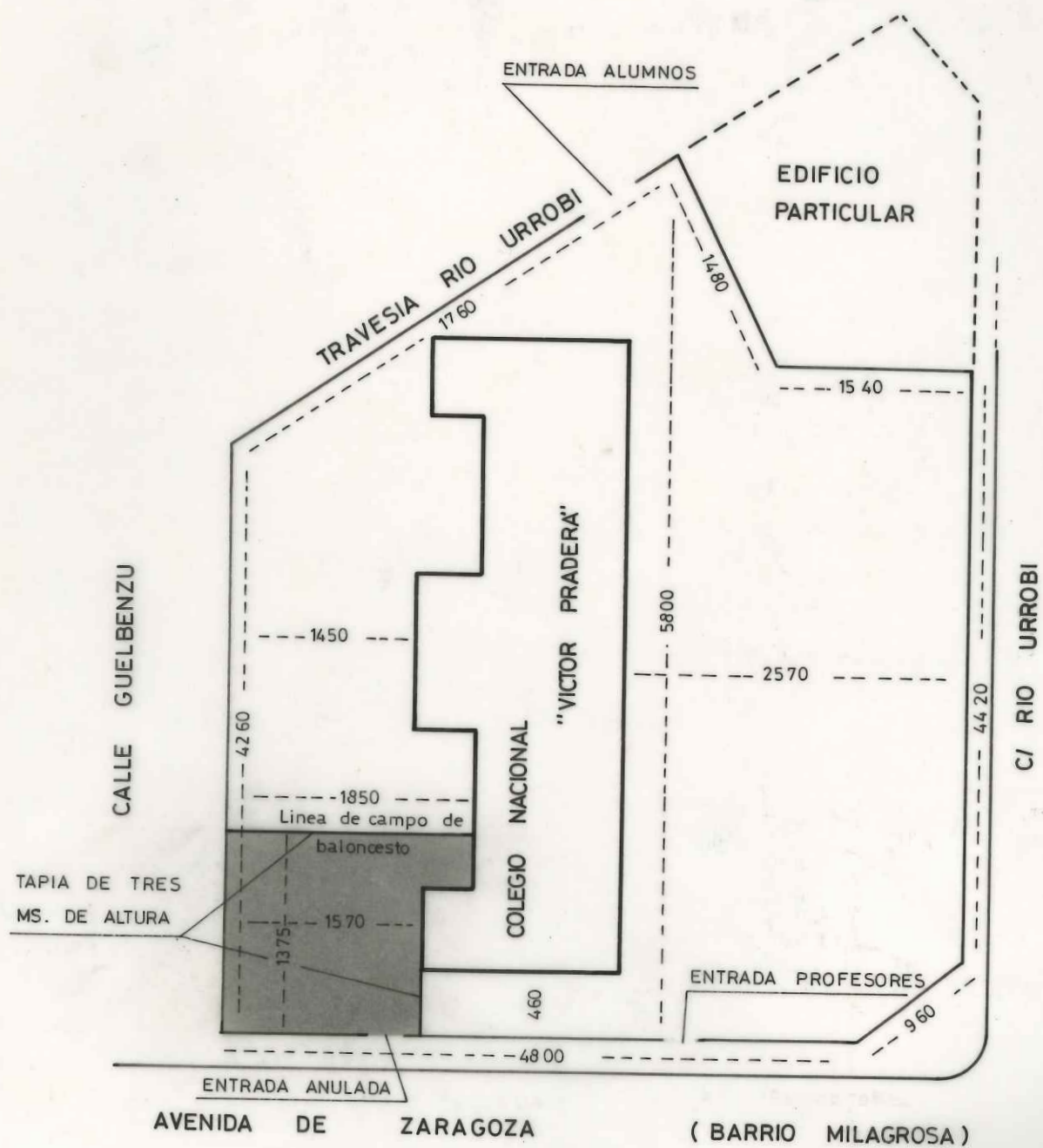
PLANTA DEL EDIFICIO Y PATIOS DEL COLEGIO NACIONAL VICTOR PRADERA DE PAMPLONA NAVARRA
