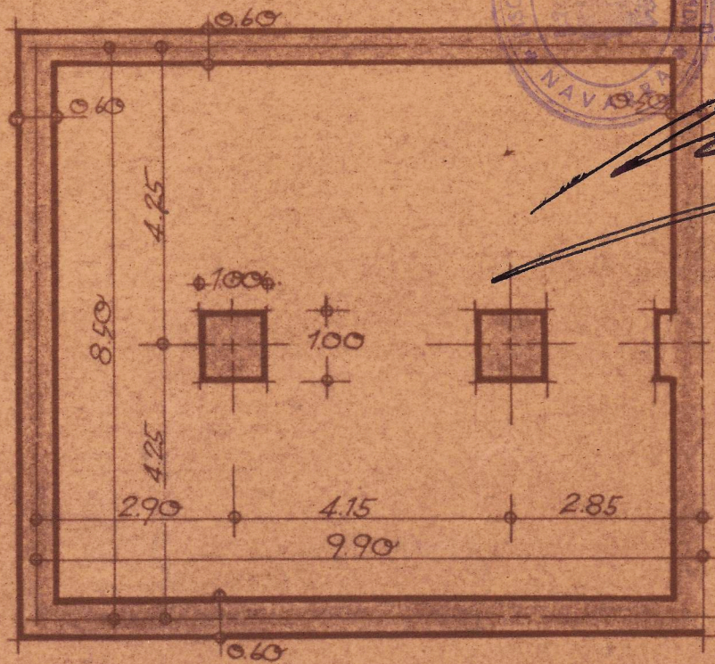
planta cimientos
