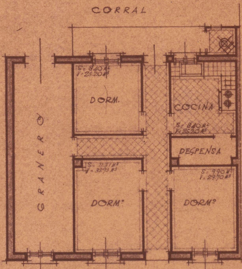
planta
