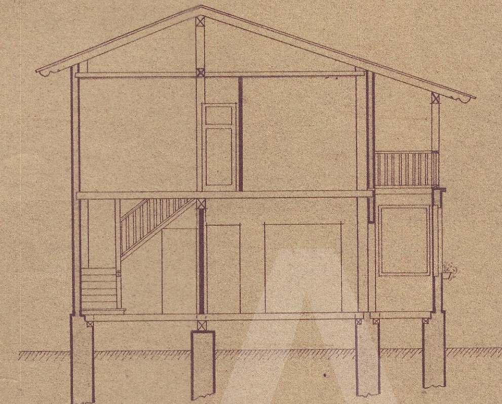
: SECCION: A.B.:
