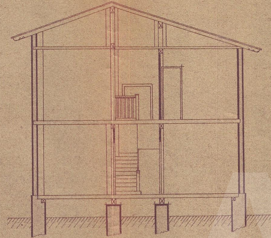
SECCION A.B.
