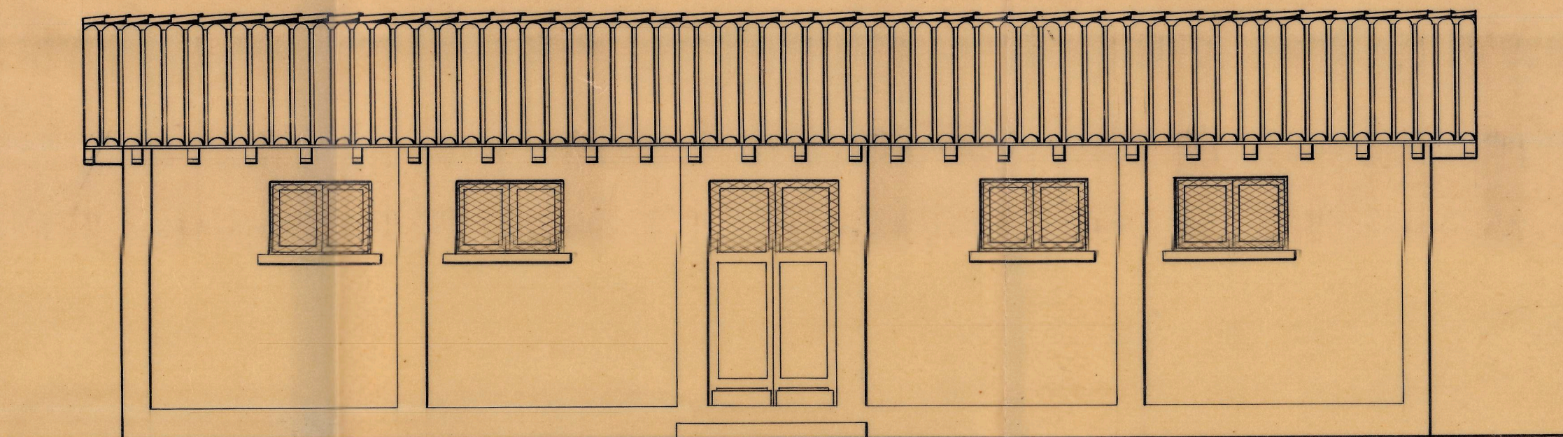
Caseta vestuario - Alzado
