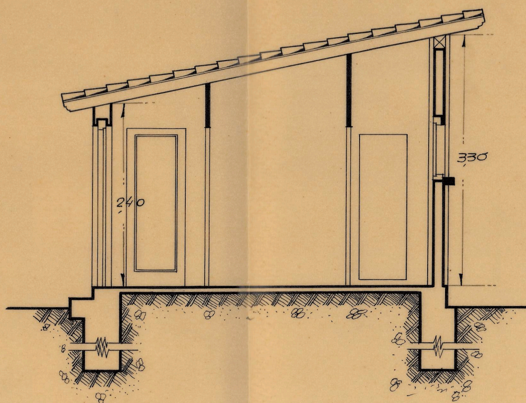
Sección a-b
