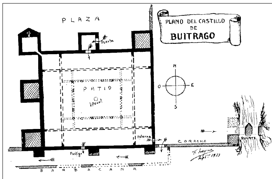
Planta del castillo de Buitrago de Lozoya (Layna Serrano, 1935).
